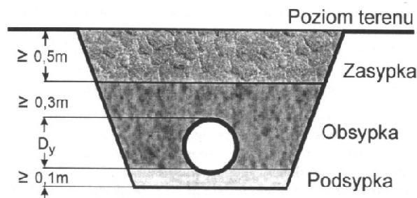
Rys. 9. Przekrój wykopu
